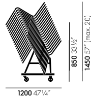
.03 chariot d'empilage
